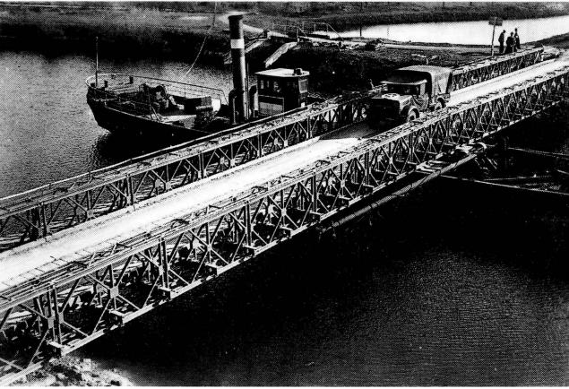
■ m.s. "Scheldestroom" als ponton voor de baileybrug ter hoogte van de Oelerbrug
